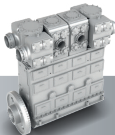
Laby® compressor
